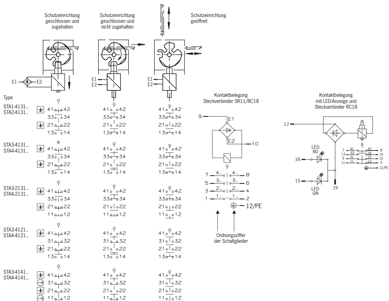
Bild 3: Schaltelemente und Schaltfunktionen
