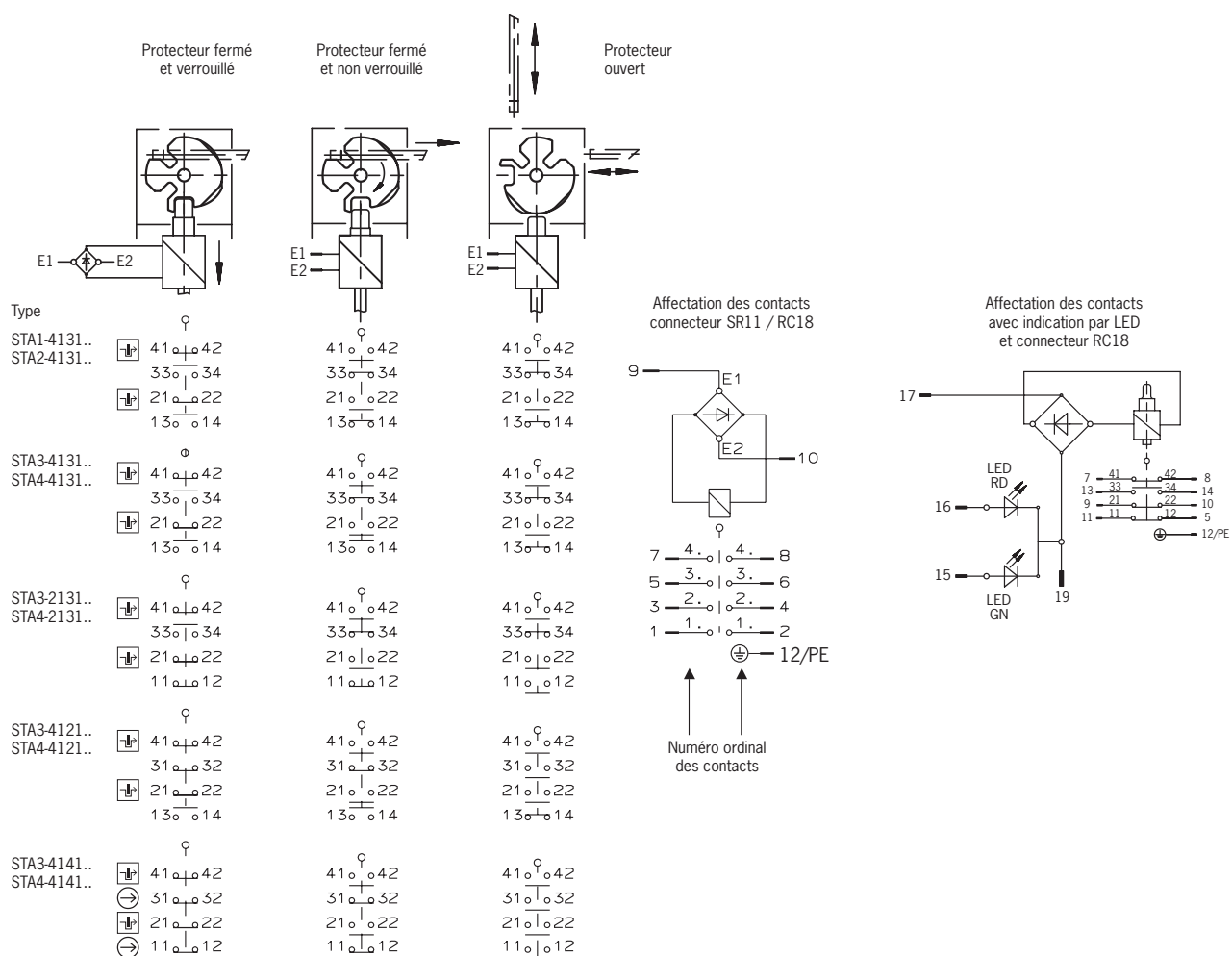
Fig. 3 : Éléments de commutation et fonctions de commutation
