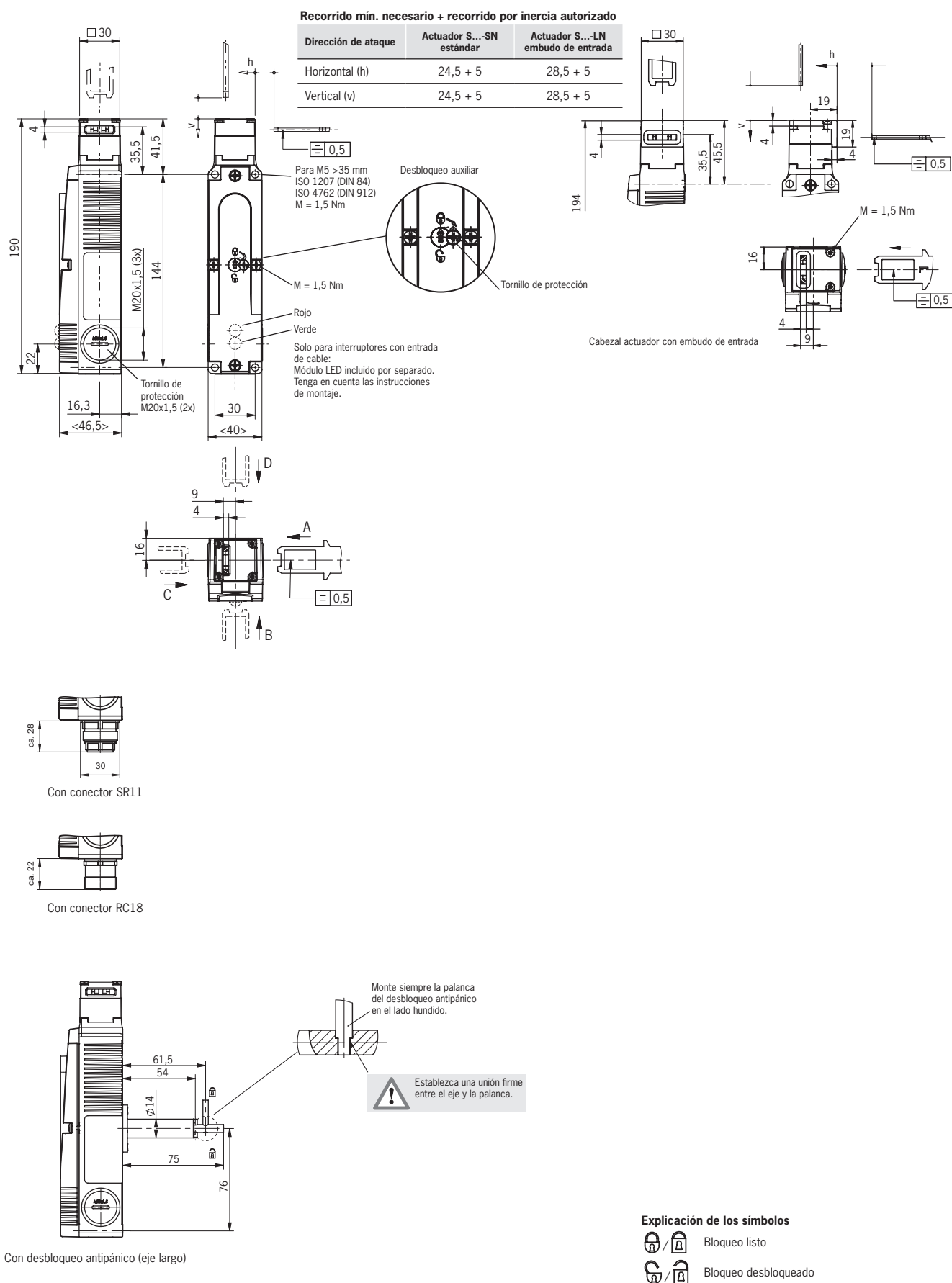
Fig. 2: Plano de dimensiones STA... sin embudo de entrada y STA... con embudo de entrada
