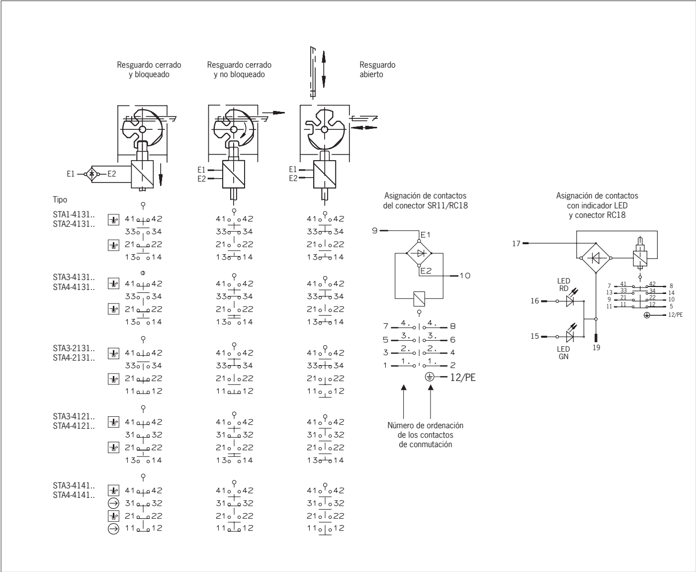
Fig. 3: Elementos interruptores y funciones de conmutación
